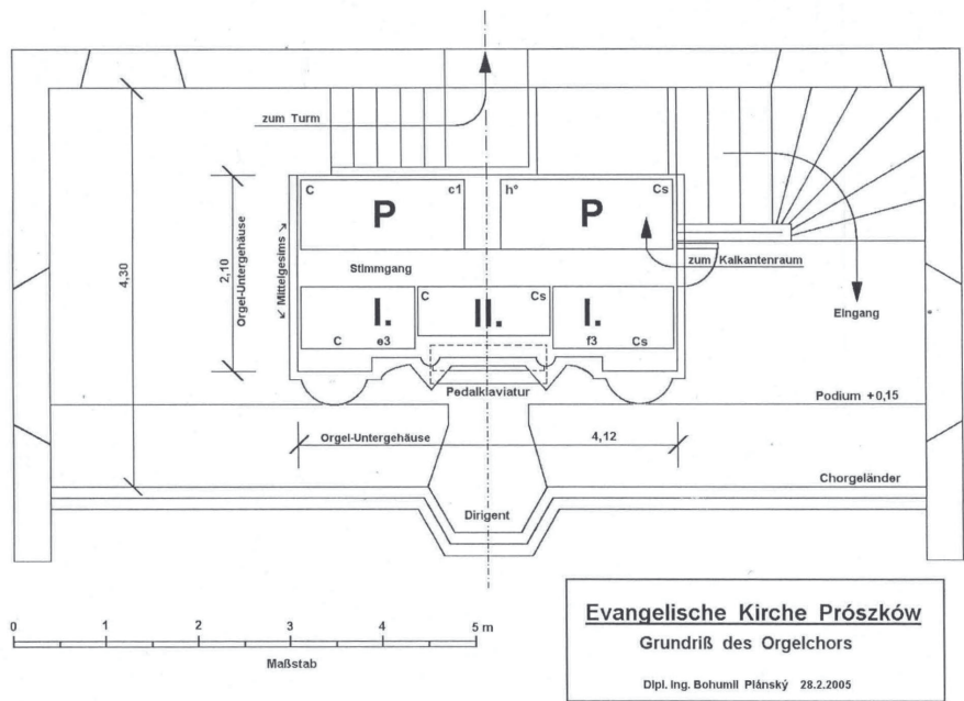
Rzut chóru muzycznego wraz z organami
